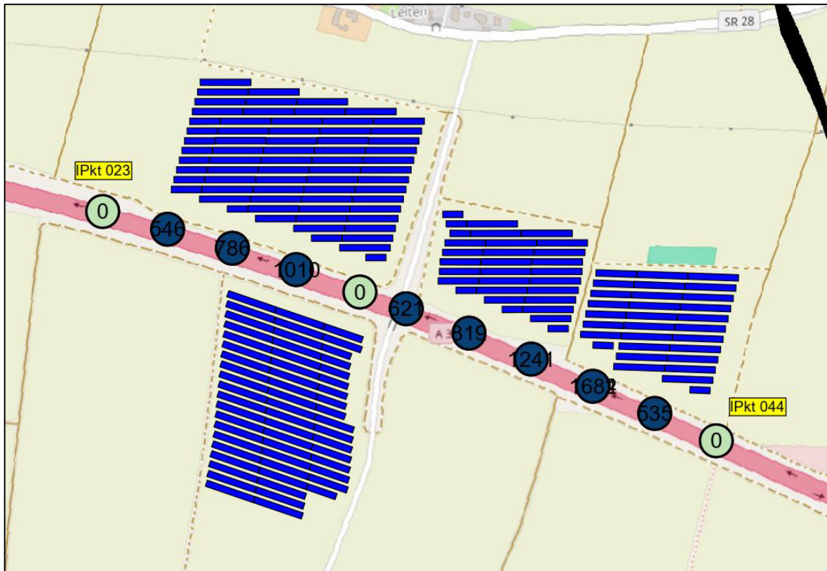
Abbildung 3: Ergebnisse der Autobahn A 3 (Fahrtrichtung West)
