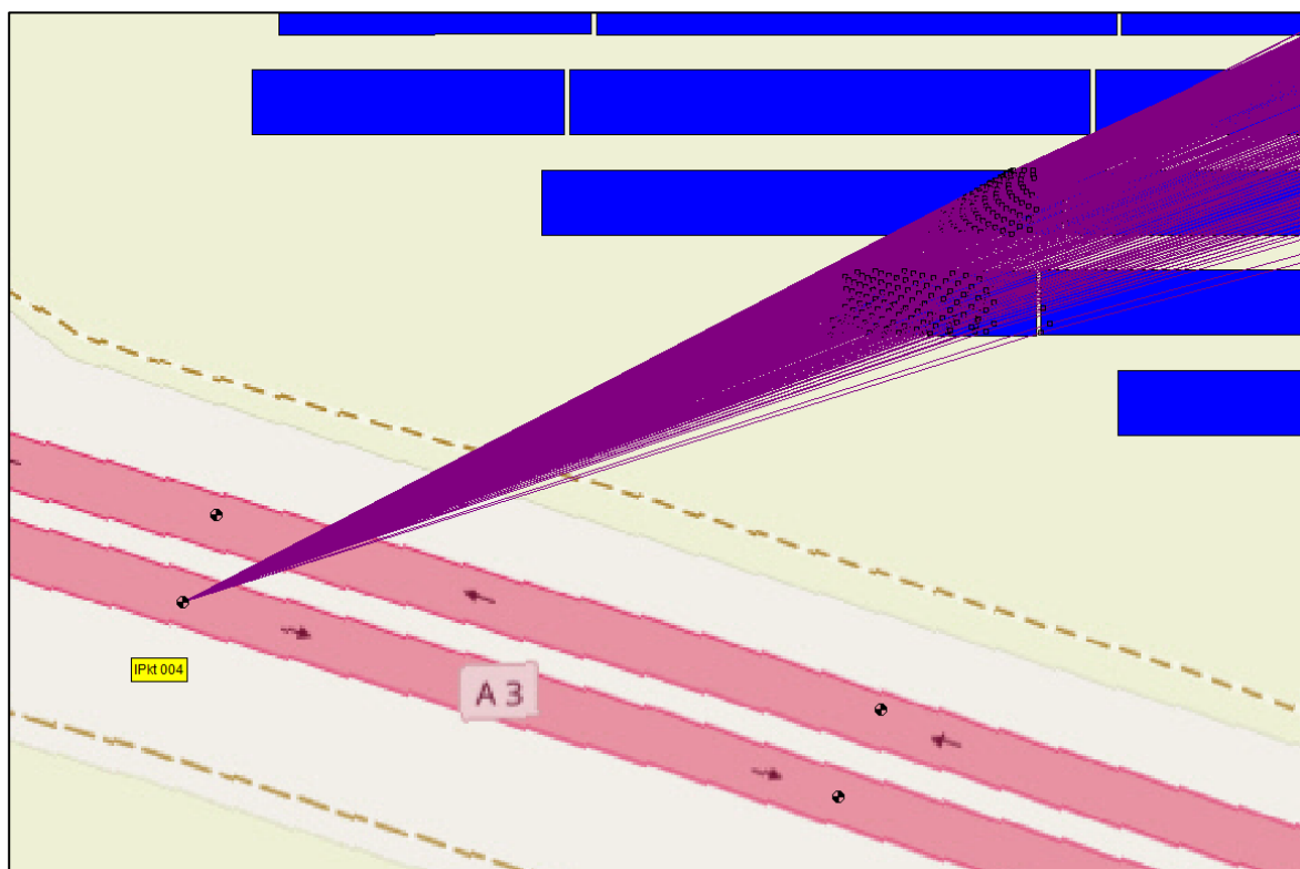
Abbildung 2: Darstellung der Reflexionen auf IPkt 004
